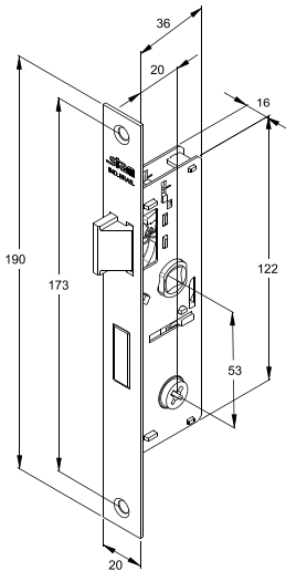
TETRA EXTERNA Máquina 600
